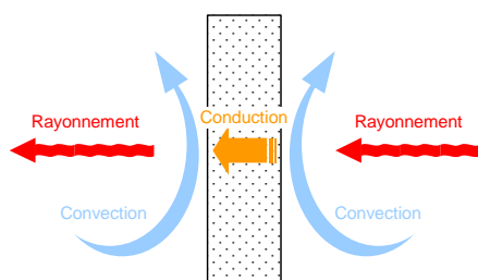
Rayonnement, convection et conduction sur une paroi
