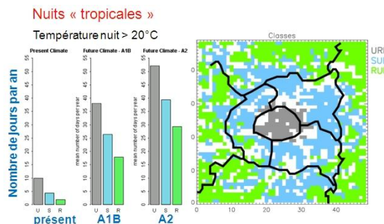
Différence de température milieux urbain / rural
