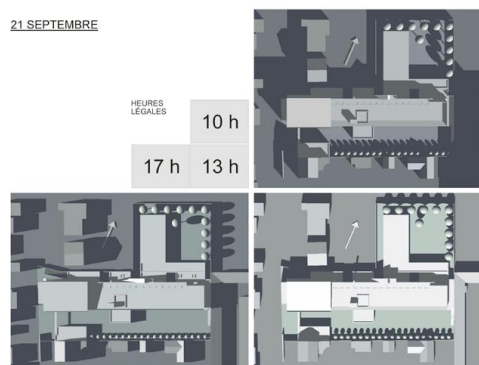
Etude des ombres portées du bâtiment sur les espaces extérieurs
